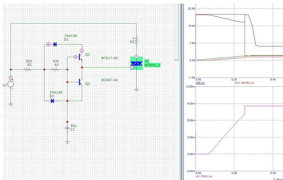
Рис. 16.2. Принципиальная схема устройства защиты громкоговорителя на тиристоре
